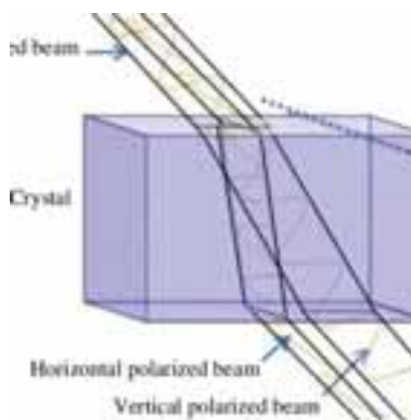
kalcitni kristal.
