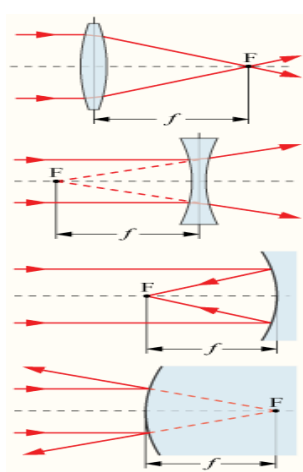
Slika 7: Lom svjetlosti kroz konvergentnu i divergentnu leću, https://tomislavdekovic.iz.hr/teorija-fotografije/
