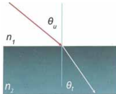
Slika 2. Zakon refrakcije.
