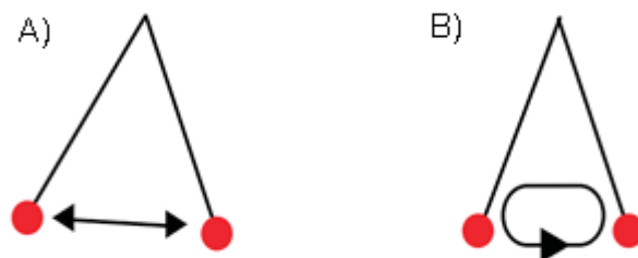
Slika7. Kretanja njihala. A) Gibanje njihala u ravnini B) Gibanje njihala u obliku elipse
