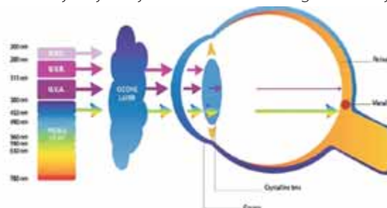
Slika 2. Apsorpcija i transmisija sunčevog zračenja u očima.
