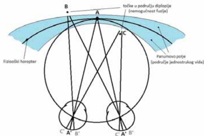
Slika 1. Vieth-Müllerov krug.
