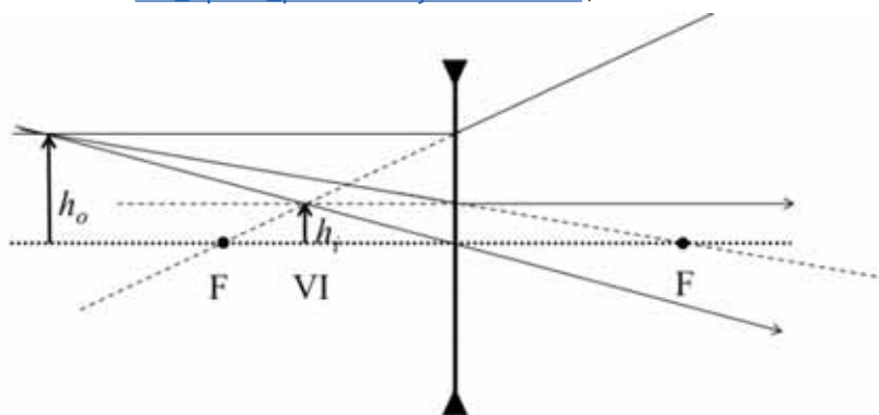
Slika 4. Karakteristične zrake svjetlosti za konkavnu leću http://phy.grf.unizg.hr/media/download_gallery/4%20F2_geometrijska_optika_preslikavanje%20lomom , 27.5.2021.
