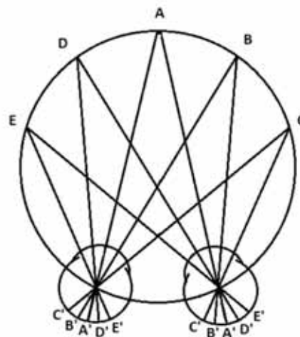
Slika 2. Fiziološki horopter.
