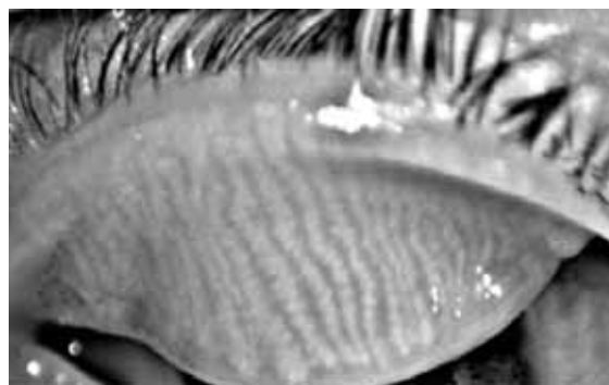
Slika 2. Meibomove žlijezde.
