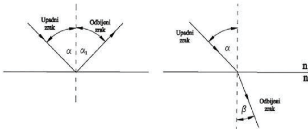
Slika 1. Zakon refleksije.
