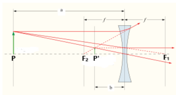
Slika 5. Nastanak slike na bikonkavnoj leći.
