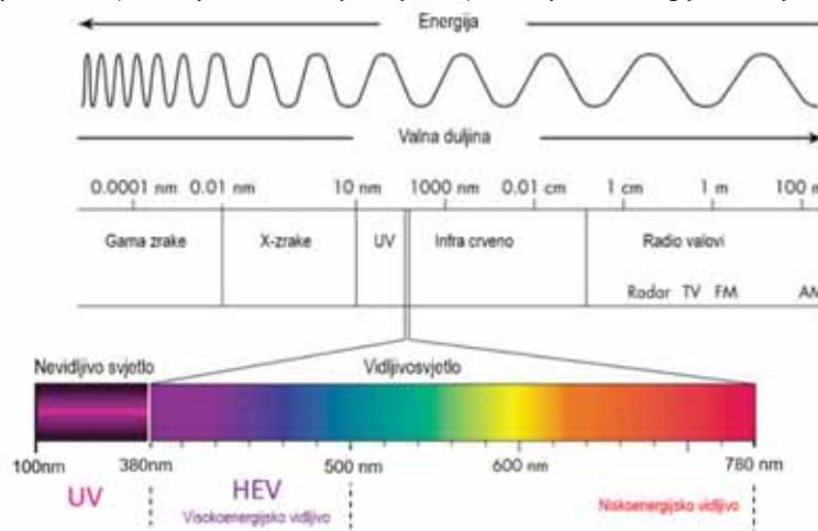
Slika 1. Raspon elektromagnetskog zračenja.
